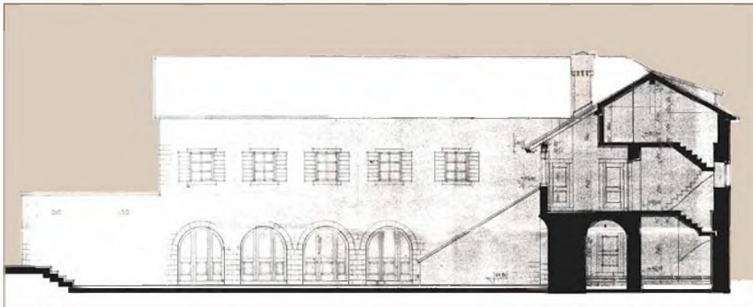
Изглед и попречни пресјек конака по конзерваторском пројекту
