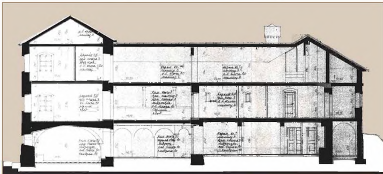
Подужни пресјек конака по конзерваторском пројекту
