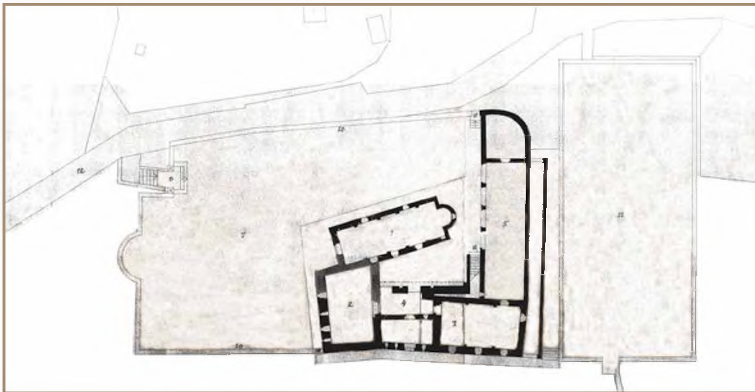
Ситуациони план манастирске порте прије реализације западног конака
